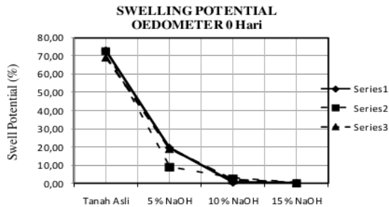
Gambar 10. Hubungan persentase campuran dengan nilai swelling potential (0 hari)
