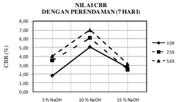
Gambar 19. Hubungan persentase campuran dengan nilai CBR (7 hari) dengan perendaman
