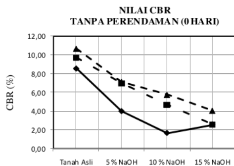
Gambar 16. Hubungan persentase campuran dengan nilai CBR (0 hari) tanpa perendaman
