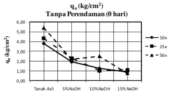
Gambar 2. Hubungan persentase campuran dengan nilai q_u (0 hari) tanpa perendaman
