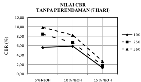
Gambar 18. Hubungan persentase campuran dengan nilai CBR (7 hari) tanpa perendaman
