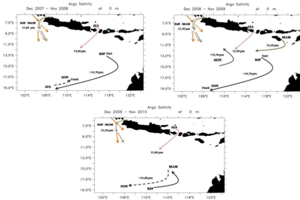
Gambar 1. Skematik distribusi salinitas permukaan secara horizontal (Lintang 5°LS- 20°LS, Bujur 100°BT-125°BT) Tahun 2004 - 2010
