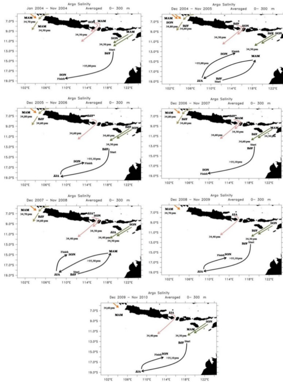
Gambar 2. Skematik distribusi salinitas secara horisontal kedalaman rerata 0-300 meter (Lintang 5°LS-20°LS, Bujur 100°BT-125°BT) Tahun 2004 - 2010
