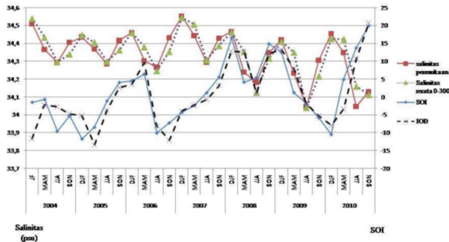
Gambar 3. Salinitas Permukaan, Salinitas Kedalaman Rerata 0 – 300 meter, Indeks SOI, Indeks IOD Tahun 2004 – 2010
