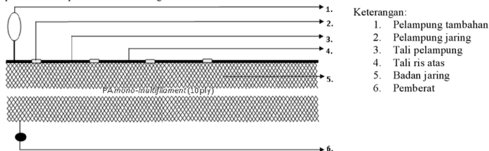
Gambar 1. Konstruksi Gillnet Millenium
