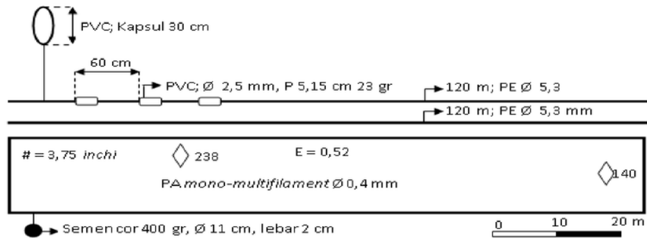
Gambar 3. Desain Gillnet Millenium
