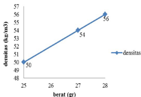
Gambar 3. Grafik hubungan nilai densitas dengan berat Foam Polyurethane
