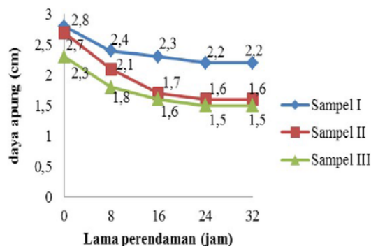
Gambar 2. Grafik Hasil Uji Apung Foam Polyurethane
