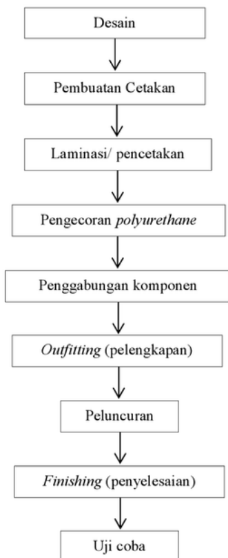
Gambar 1. Diagram Alir Proses Pembuatan Kapal Ikan Fiber
