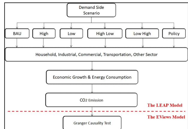
Fig. 1. Framework Scenario
