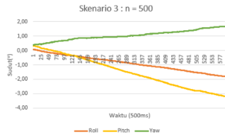
Gambar 9. Hasil pengujian Skenario 3 dengan n =500
