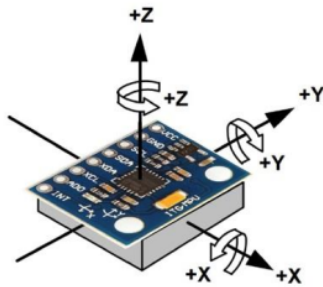
Gambar 4. Orientasi aksis pada sensor MPU-6050
