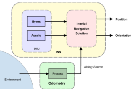
Gambar 1. Integrasi IMU-Odometri untuk menghasilkan informasi navigasi
