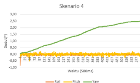
Gambar 10. Hasil pengujian Skenario 4
