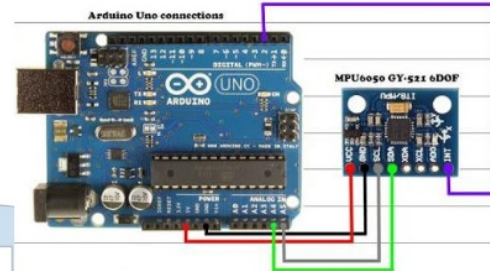
Gambar 2. Diagram wiring antara Arduino Uno dan MPU 6050
