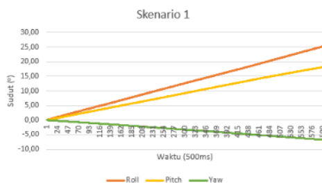
Gambar 5. Hasil pengujian Skenario 1
