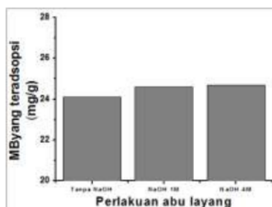
Gambar 2. Hubungan antara MB yang teradsorpsi oleh abu layang baik tanpa dan dengan perlakuan dengan NaOH untuk menyerap 50 mL MB 50 mg/L.
