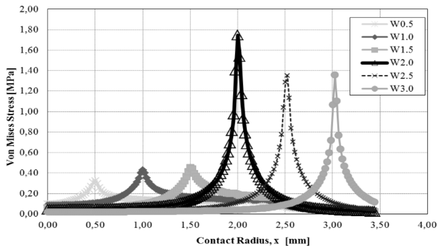
Gambar 7. Distribusi tegangan von Mises sebagai fungsi dari jari-jari kontak dengan variasi jari-jari celah yang diberikan pada material UHMWPE sebagai acetabular liner .
