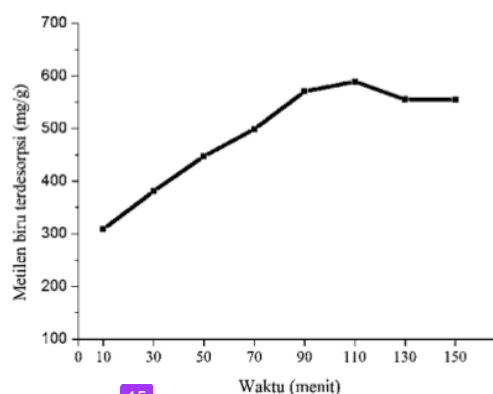
Gambar 9. Pengaruh waktu kontak terhadap metilen biru yang terdesorpsi
