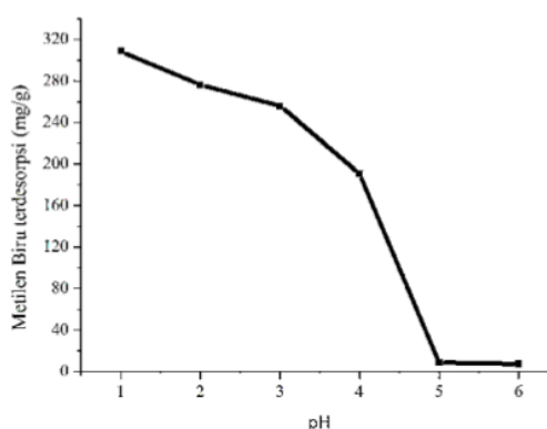
Gambar 8. Pengaruh pH terhadap metilen biru yang terdesorpsi
