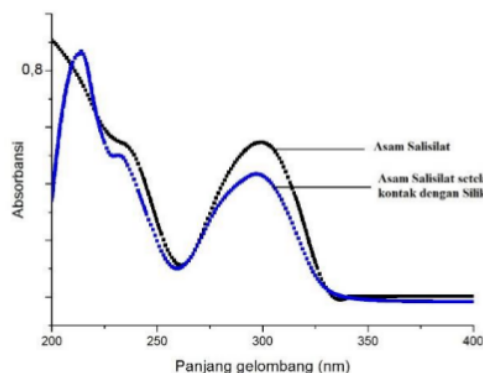
Gambar 4. Spektra UV-Vis asam salisilat dan asam salisilat setelah kontak dengan silika
