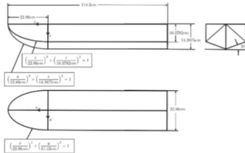
Gambar 1. Persamaan garis pada Fridsma hull form
