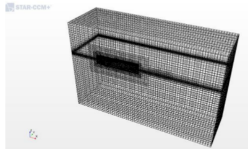
Gambar 5. Ilustrasi konfigurasi kerapatan mesh
