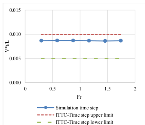
Gambar 3. Penggunaan time-step CFD
