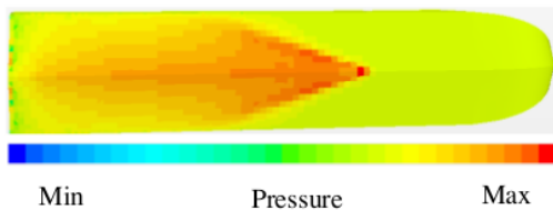
Gambar 7. Perbedaan pressure pada saat simulasi CFD
