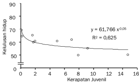
Gambar 11. Hubungan kerapatan juvenil (ind.100 cm -2 ) dengan kelulusan hidup juvenil karang P. damicornis yang menempel pada substrat penempelan di Pulau Panjang
