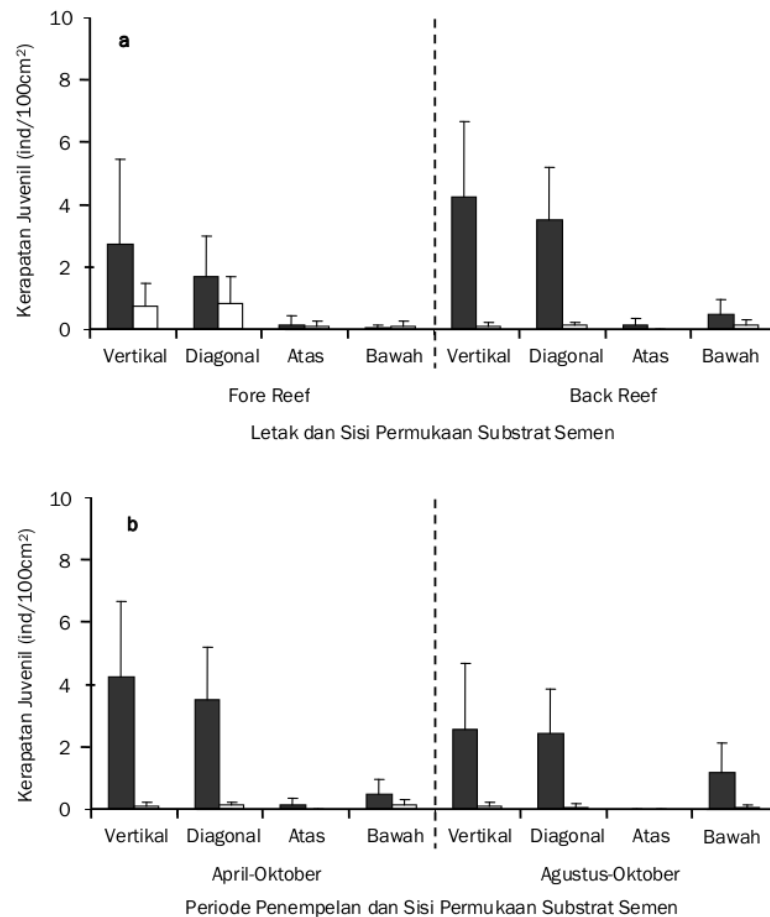
Gambar 6. Kerapatan juvenil karang P. damicornis di P. Panjang pada berbagai sisi permukaan substrat semen (a. Letak substrat; b. Periode penempelan). Keterangan : □ = Utara, ■ = Selatan
