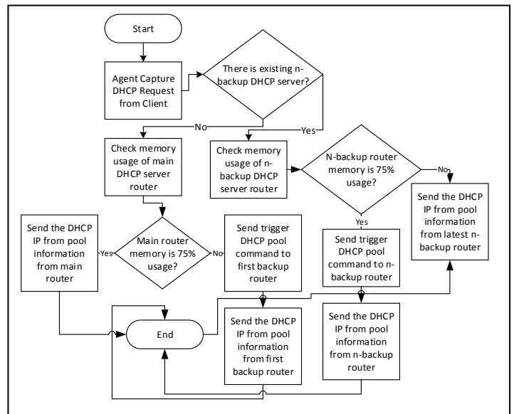
Fig. 3. DHCP Centralization Scenario.
