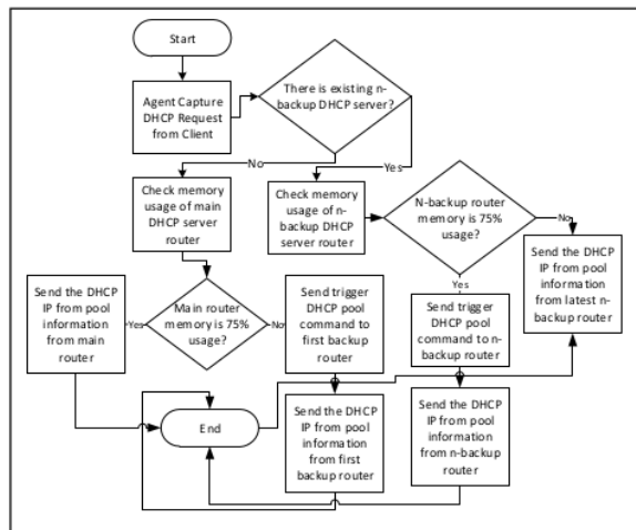
Fig. 3. DHCP Centralization Scenario.
