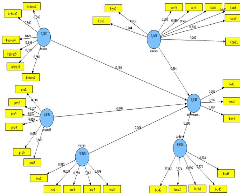
Gambar 2 Output Perhitungan Menggunakan PLS
