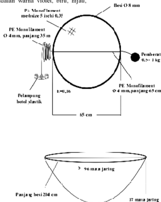
Gambar 1. Desain Alat Tangkap Krendet
