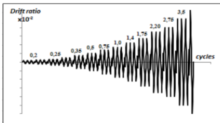
Gambar 6. Urutan Siklus Pembebanan (ACI 374.1-05)
