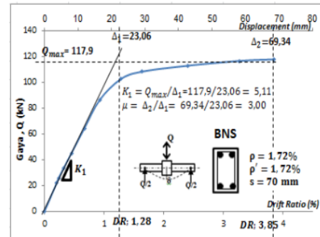
Gambar 11. Kurva envelope perilaku spesimen BNS
