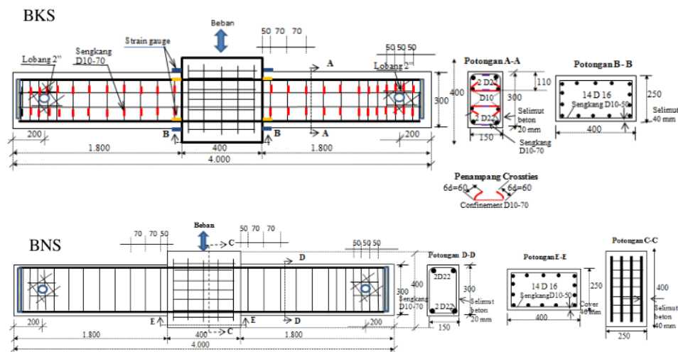
Gambar 2. Benda uji BKS dan BNS
