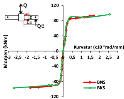
Gambar 12. Kurva envelope dua arah BKS dan BNS
