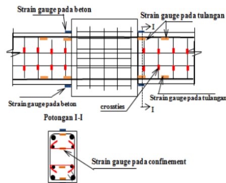
Gambar 3. Instrumentasi pada spesimen.
