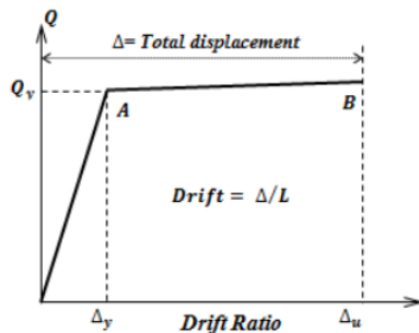
Gambar 5. Deformasi komponen (ACI 374.1-05)
