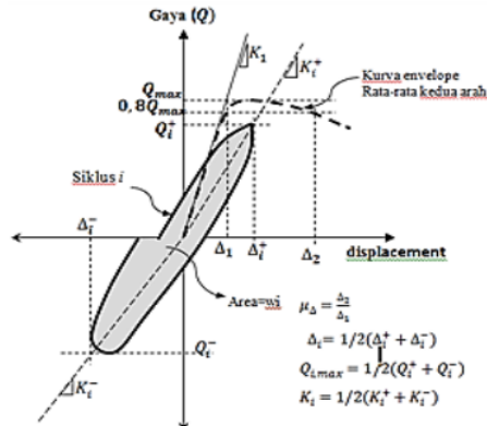
Gambar 9. Parameter daktilitas (Bayrak & Sheikh, 1998)
