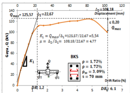
Gambar 10. Kurva envelope perilaku spesimen BKS
