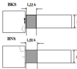
Gambar 8. Wilayah kerusakan BKS dan BNS
