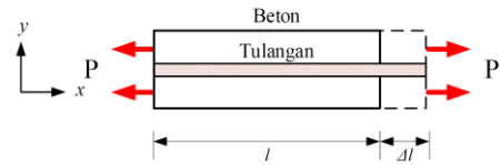
Gambar 8. Dasar teori kompatibilitas beton-tulangan
