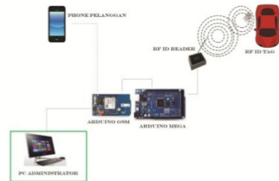
Gambar 1. Arsitektur purwarupa Sistem GTO ramah lingkungan berbasis RFID yang diusulkan.
