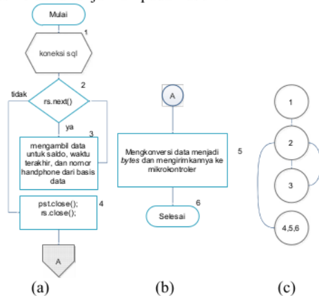
Gambar 4. Fungsi mengirim SMS pada halaman utama User Admin , (a) Flowchart mengambil data() , (b) Flowchart kirimdatastring() , dan (c) Flowgraph
