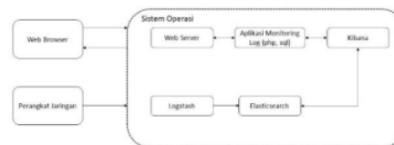
Gambar 2. Desain Sistem Server
