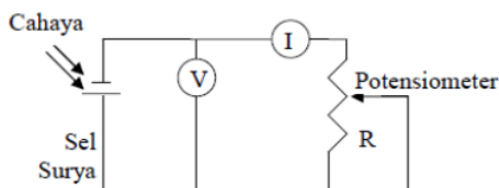
Gambar 2. Skema rangkaian listrik pengujian sel surya
