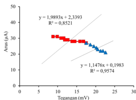
Gambar 12. Kurva I-V Sel Surya pada ZnO B (dengan PVA)
