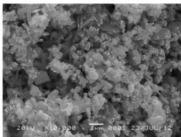
Gambar 9. Morfologi permukaan lapis tipis ZnO A dan metode doctor blade dengan perbesaran 10.000 x
