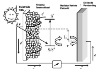
Gambar 1. Skema prinsip sel surya fotoelektrokimia tersensitisasi dye
