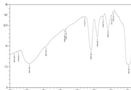
Gambar 7. Spektra inframerah lapis tipis ZnO B dengan zat warna
