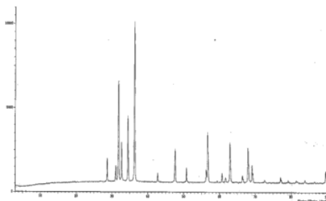
Gambar 5. Difraktogram Lapis Tipis ZnO B (PVA) pada substrat kaca
