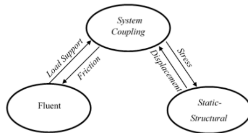
Gambar 1. Teknik fluid-structure interaction (FS) pada perangkat lunak
