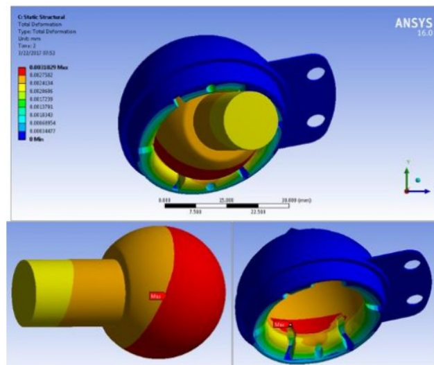
Gambar 7. Kontur deformasi pada artificial hip joint
