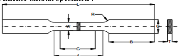
Gambar 5. Bentuk Spesimen [7]
