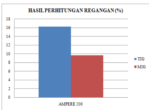
Gambar 9. Grafik Rata-rata Regangan
