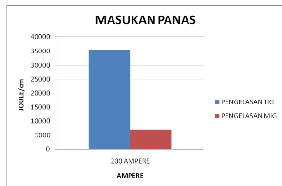
Gambar 7. Grafik masukan panas ( Heat Input )
