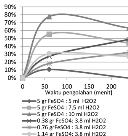
Gambar 4. Persentase Penyisihan BOD pada proses Fenton
