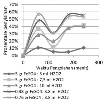
Gambar 3. Persentase Penyisihan COD pada proses Fenton
