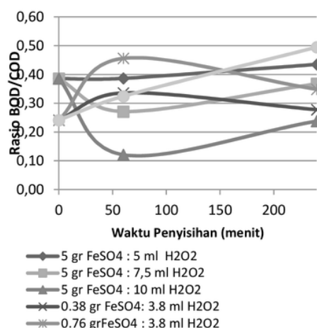
Gambar 5. Perubahan Rasio BOD/COD sebelum dan sesudah proses Fenton
