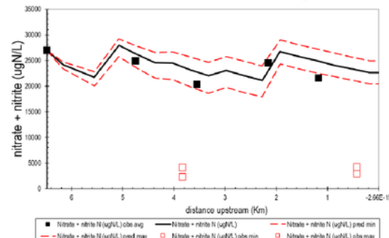
Gambar 8. Hasil Pemodelan Nitrat Eksisting
