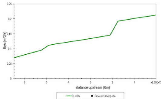
Gambar 5. Hasil Pemodelan Debit Eksisting
