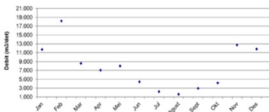
Gambar 4. Prkiraan Debit di Sungai Anyar yang digunakan untuk suplesi Sungai Pepe Sumber : Dinas Lingkungan Hidup Kota Surakarta 2017
