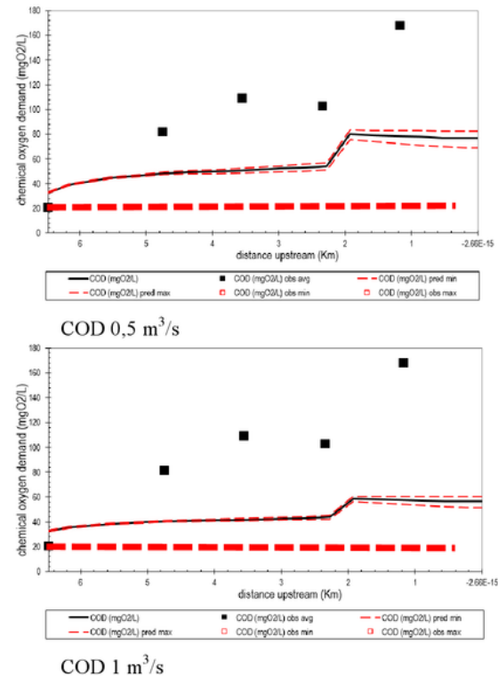
Gambar 10. Hasil Pemodelan COD
