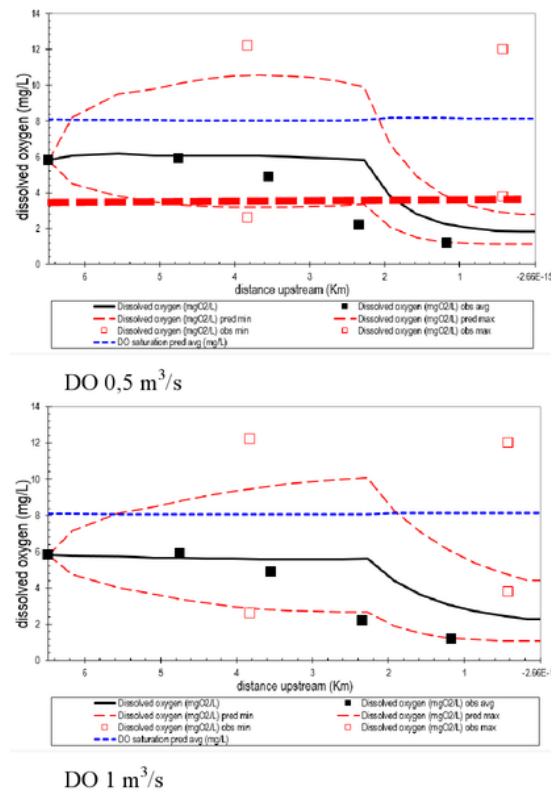
Gambar 9. Hasil Pemodelan DO
