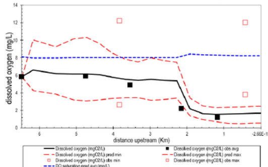
Gambar 6. Hasil Pemodelan DO Eksisting
