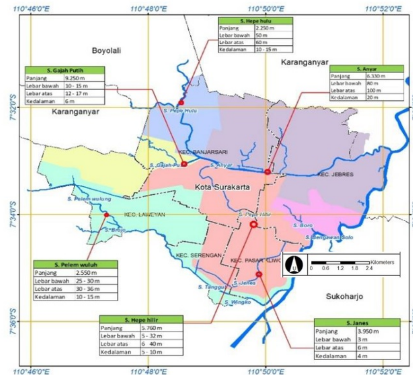
Gambar 2. Hubungan Aliran Sungai di Kota Surakarta
