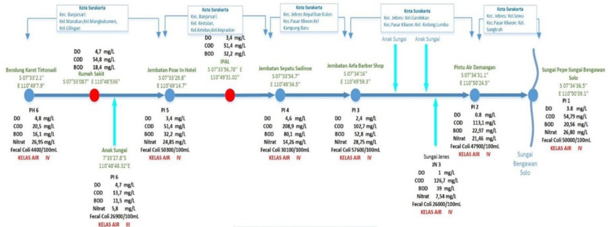
Gambar 3. Skema Titik Sampling Sungai Pepe Hilir
