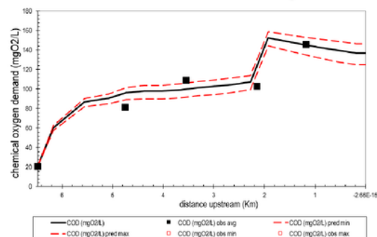
Gambar 7. Hasil Pemodelan COD Eksisting
