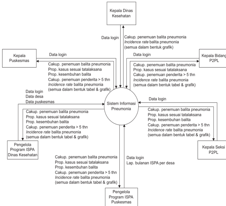
Gambar 2. Diagram Konteks SI Pelaporan Rutin Pneumonia Setelah Dikembangkan
