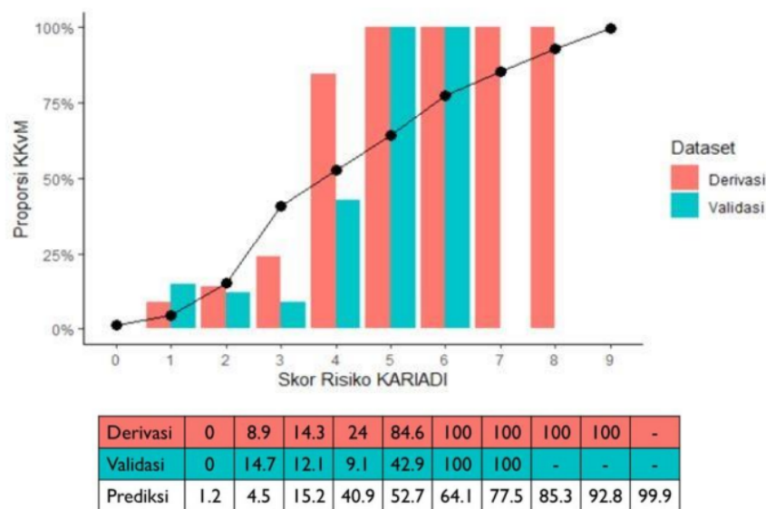
Gambar 2. Perbandingan proporsi kejadian kardiovaskular mayor yang diobservasi pada kohort derivasi dan validasi vs. prediksi
