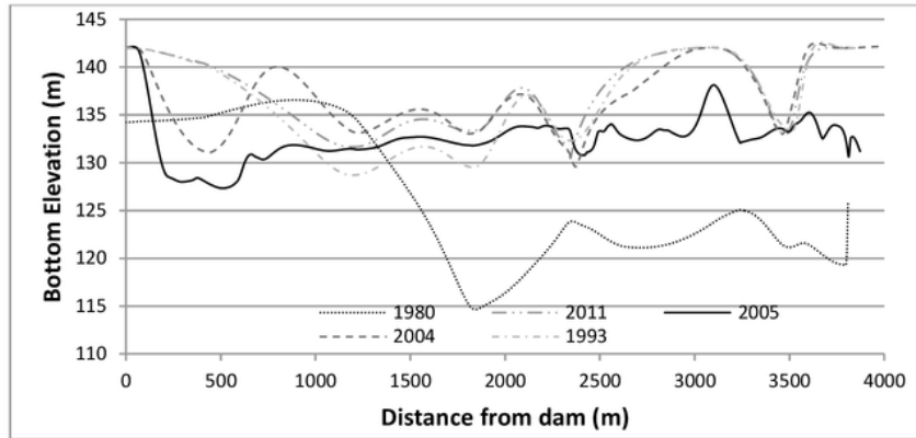
Fig. 5. Longitudinal Profil of Keduang River
