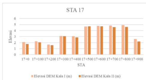
Gambar 8. Perubahan Elevasi STA 17
