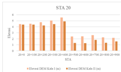
Gambar 11. Perubahan Elevasi STA 20
