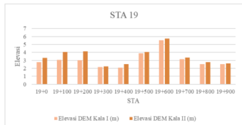
Gambar 10. Perubahan Elevasi STA 19
