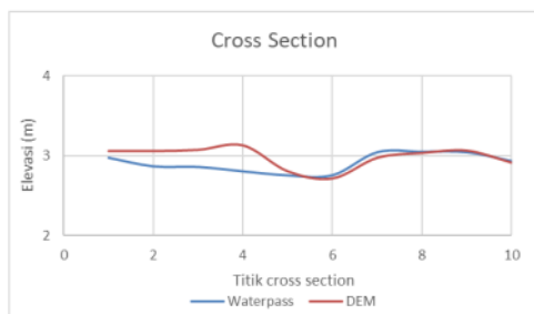
Gambar 15. Hasil Perbandingan Cross Sections dan DEM
